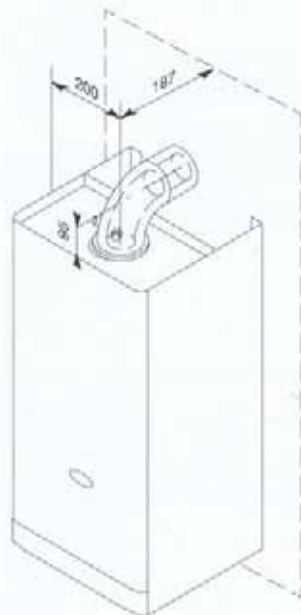
Posizione asse camino
