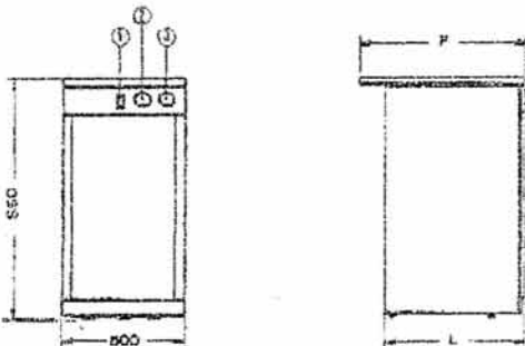
1) Interruttore Estate-Inverno - 2) Termometro caldaia - 3) Termostato priorità
