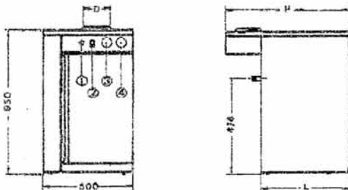
1) Termostato di sicurezza - 2) Interruttore con segnalazione - 3) Termometro caldaia - 4) Termostato di regolazione
